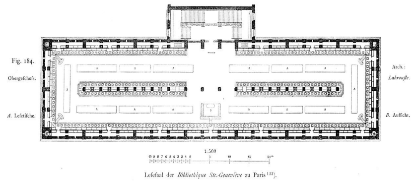
Planta principal
