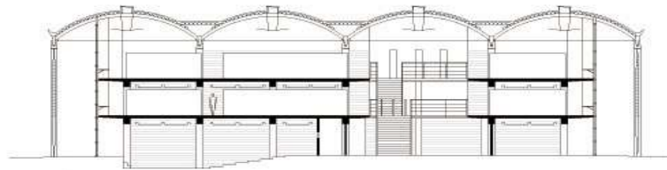
Sección AA' E. 1/300
